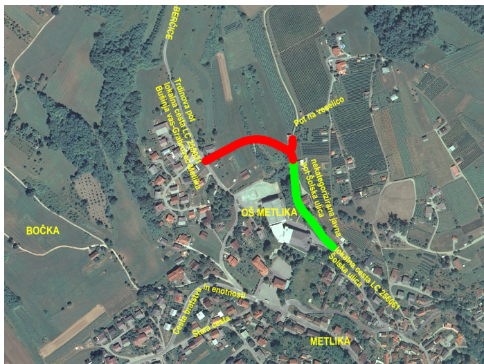
Slika: Območje izgradnje nove povezovalne ceste s pločnikom in javno razsvetljavo - 1. faza (rdeča barva) ter rekonstrukcije Šolske ulice - 2. faza (zelena barva)
